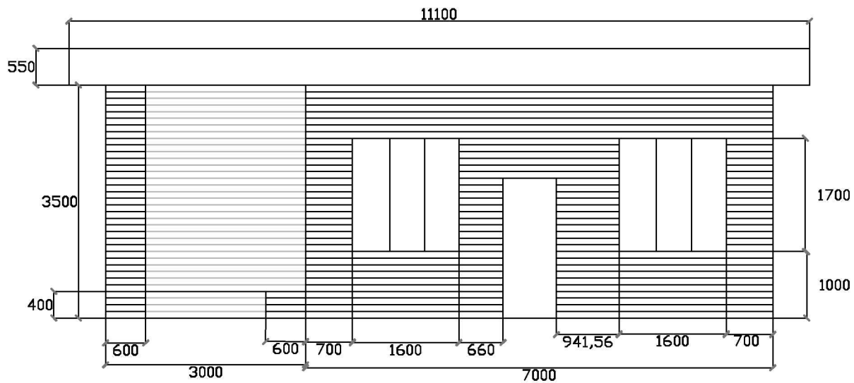
Вид спереди
