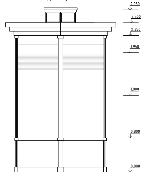
Вид сбоку
