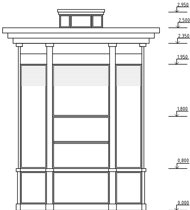
Вид спереди
