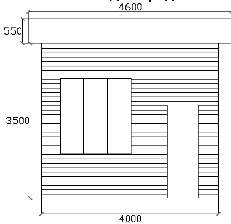
Вид спереди
