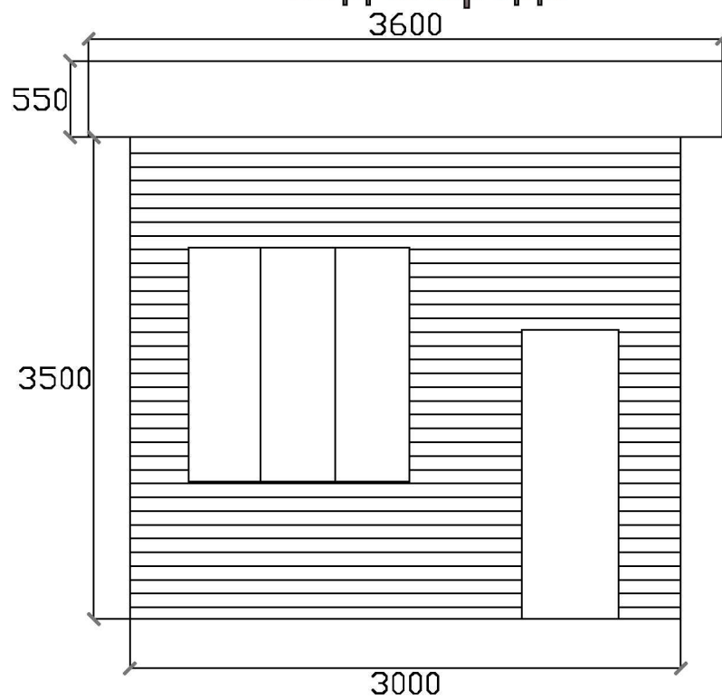
Вид спереди
