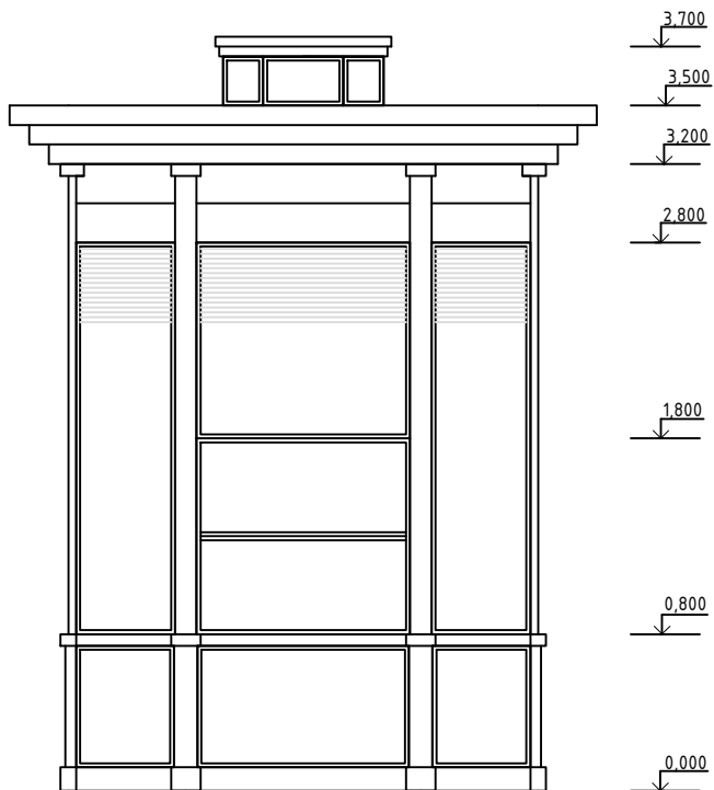
Вид спереди
