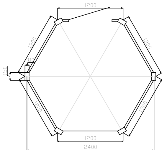
Вид сверху в разрезе
