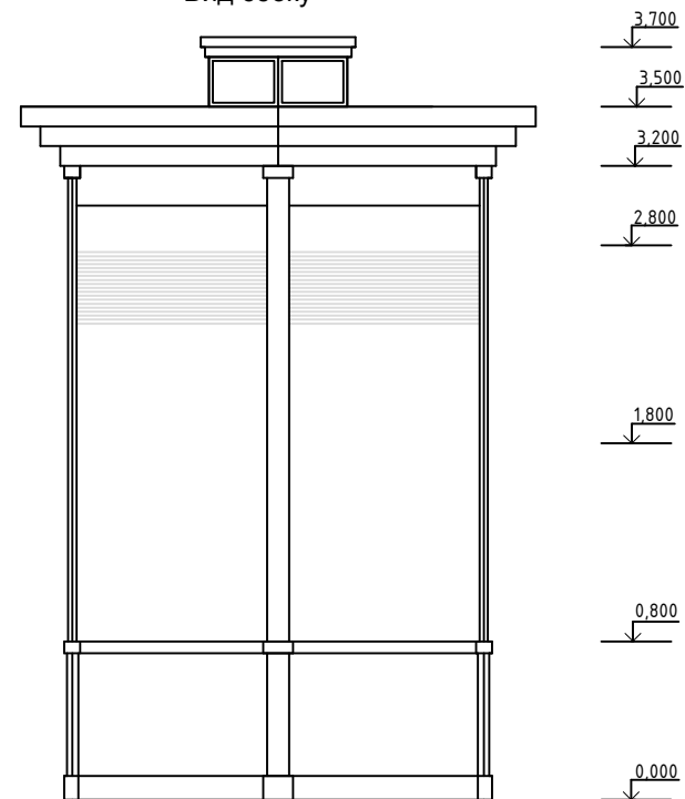
Вид сбоку
