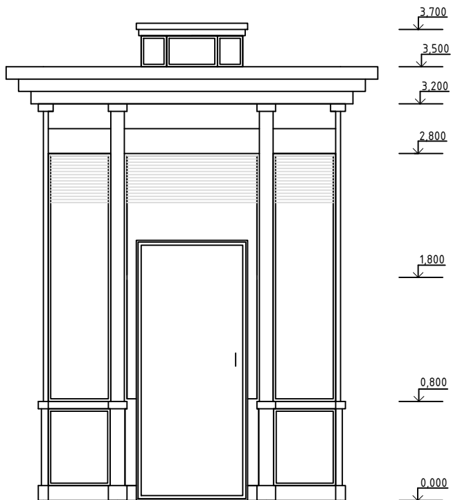
Вид сзади
